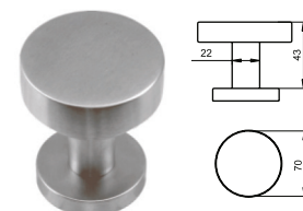
D57x70 FIXO AISI 304
