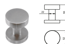
D57x55 FIXO AISI 304
