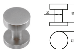
D57x55 ROT AISI 304
