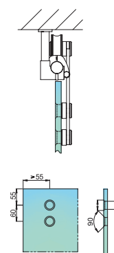
Portas de Correr Aplicação ao Tecto
