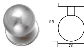
D70 FIXO AISI 304
