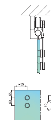
Portas de Correr Aplicação ao Tecto
