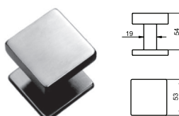
K58Dx55 FIXO AISI 304
