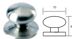
DF 85x70 AISI 304
